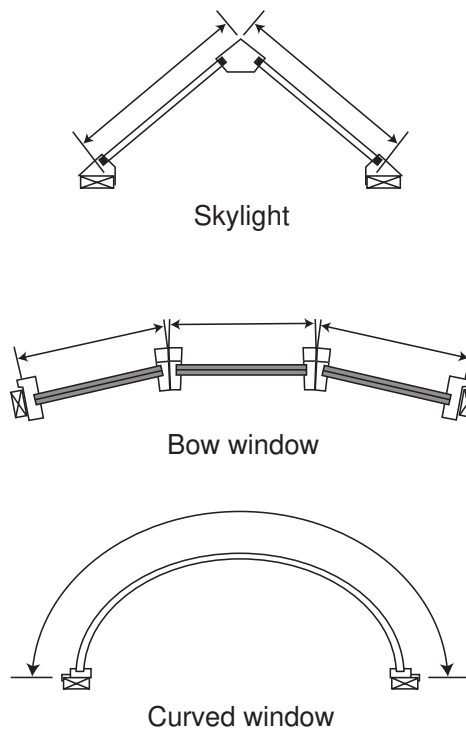
Figure A-3.1.1.6.(5)
